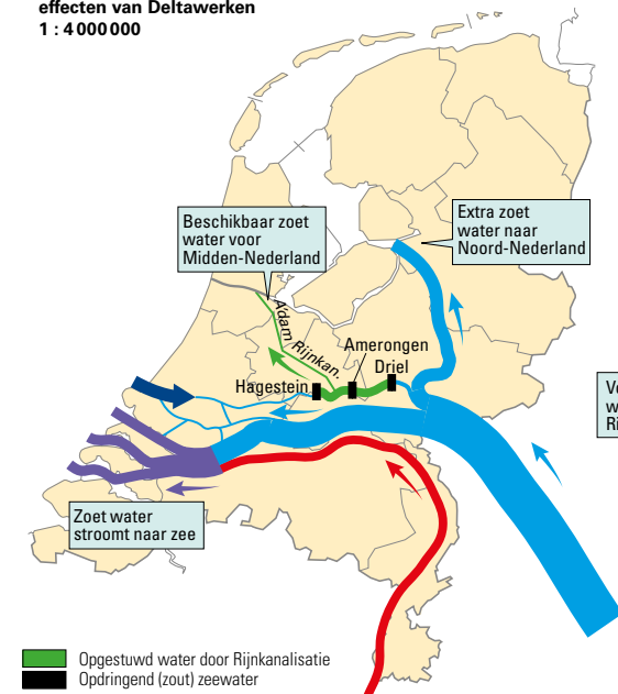
C3. Waterverdeling na Rijnkanalisatie en uitvoering Deltawerken 1 : 4 000 000
