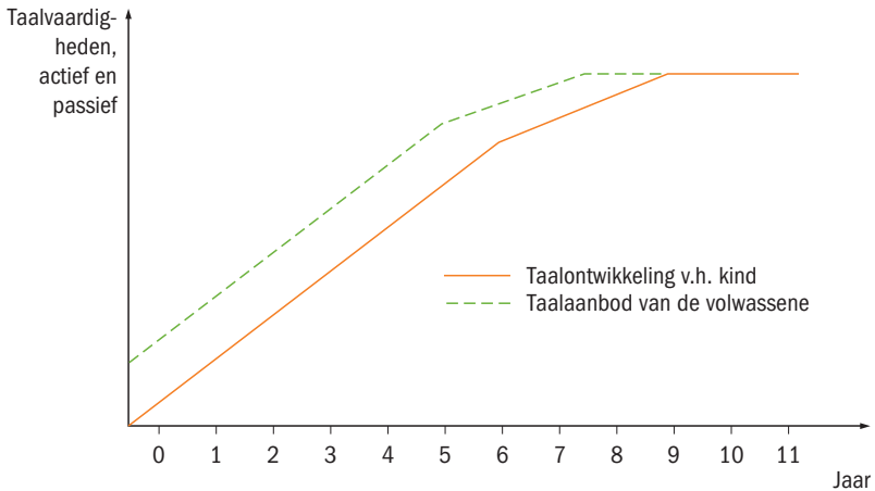
FIGUUR 1.1 Taalontwikkelingslijn
