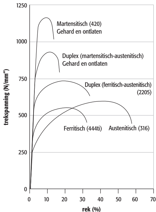
Figuur 1.14 Trekkromme van diverse roestvaststaalsoorten.
