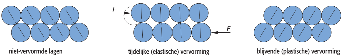
Figuur 1.13 Elastische en plastische vervorming.
