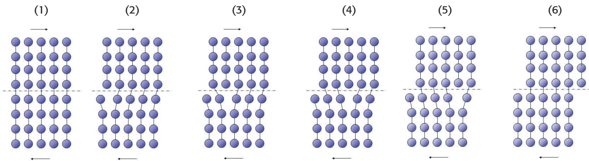
Figuur 1.10 In stappen 1 tot en met 6 worden de achtereenvolgende stappen bij het plastisch deformeren van een metaal getoond. Dit verschuiven vindt plaats op de zwakste plaats (daar waar bijvoorbeeld vacatures of dislocaties zijn). In de figuur hiernaast is een schematische afbeelding van een dislocatie die zich uit als een lijnfout.
