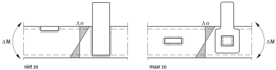
Figuur 1.2 Voorbeeld van het lassen van onderdelen daar waar het weinig kwaad kan.
