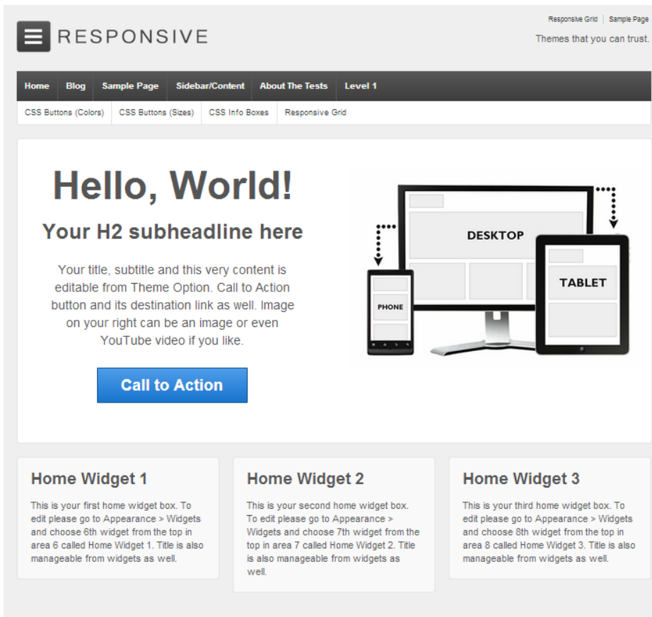
Afbeelding 3.32 –Responsive theme
