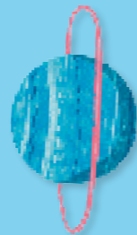
Uranus
