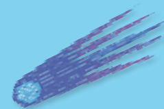
komeet
