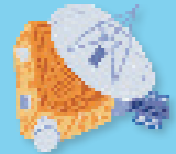
ruimtesonde
