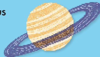
Saturnus
