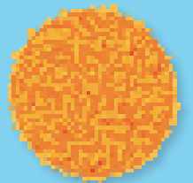
zon
