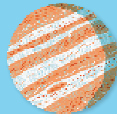
Jupiter
