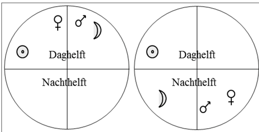
Fig. 25. De nachtplaneten in de daghelft en in de nachthelft van een daghoroskoop.
