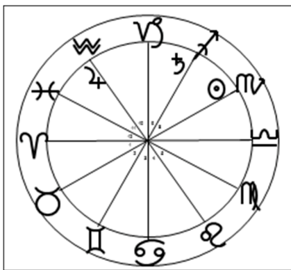
Fig. 28. Fortuinlijke sect voor de dagplaneten Jupiter en Saturnus.
