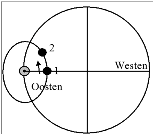
Fig. 14. Het ochtendrijzen van Venus.
