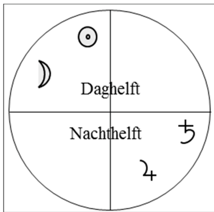
Fig. 27. Verschuiving met ca. 3 uur draaiing van de Aarde.
