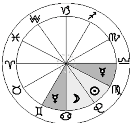
Fig. 9. De plaatsing van Mercurius naast de positie van Venus.
