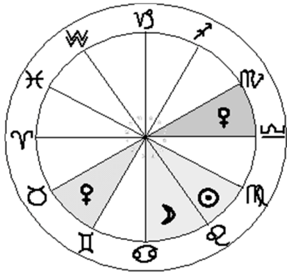
Fig. 8. De plaatsing van Venus naast de positie van Mars.
