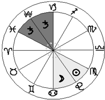
Fig.5. De plaatsing van Saturnus tegenover de tekens Kreeft en Leeuw.
