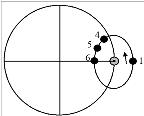
Fig.13. De ondergang van Venus in het Westen.
