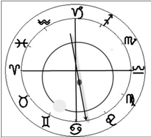
Fig. 3. Stelsel met deferent en epicykel.
