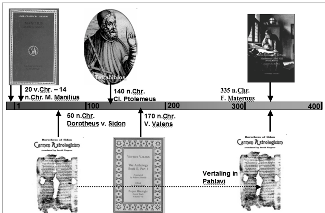
Fig. 1. Eenvoudige tijdlijn van de Hellenistische astrologie.
