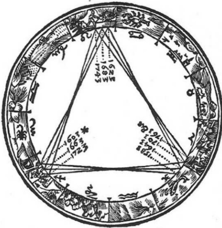
Johannes Keplers trigon, een diagram van grote voegwoorden uit het boek "De Stella Nova" (1606).
