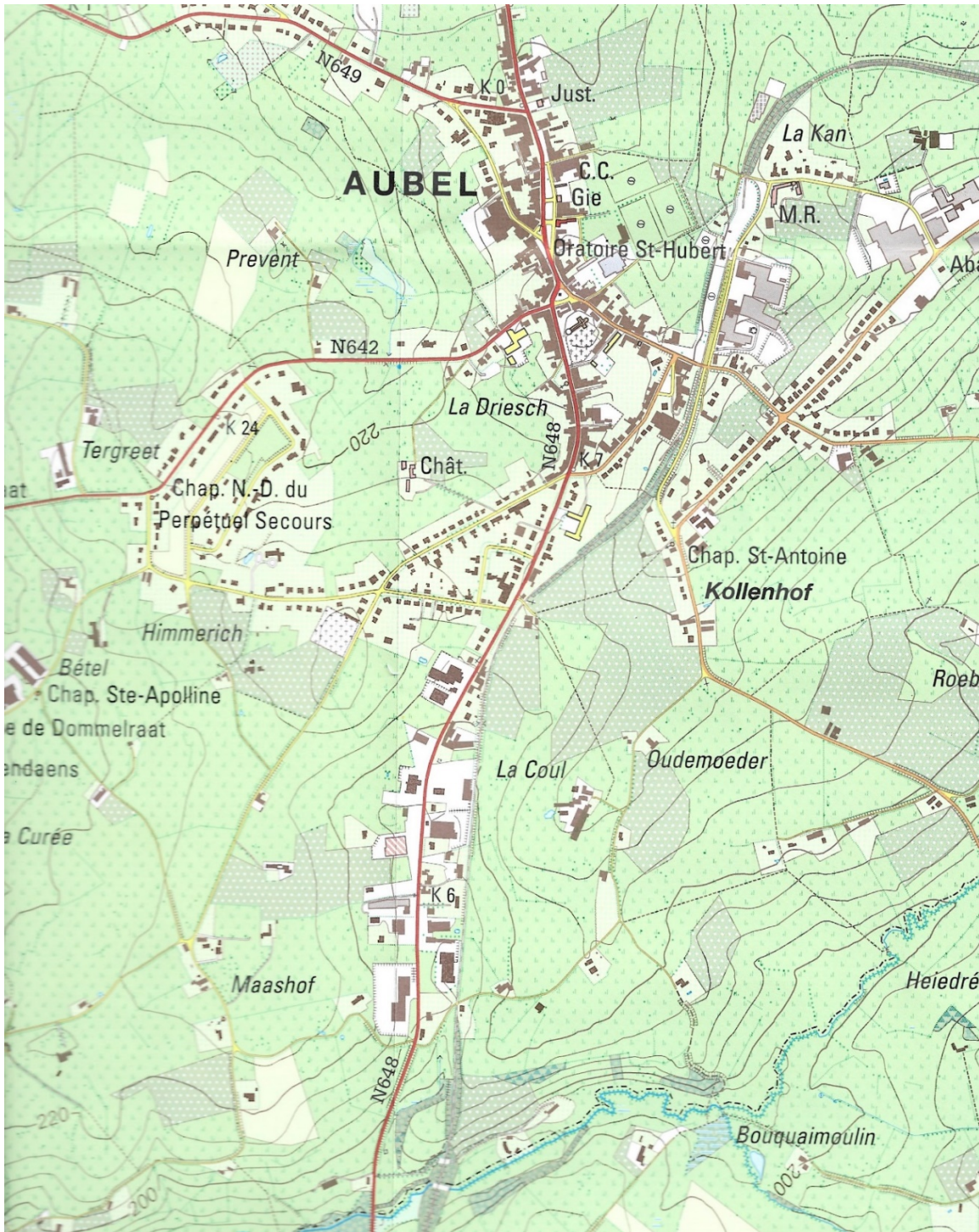
Aubel: topografische kaart, 1:10.000.
