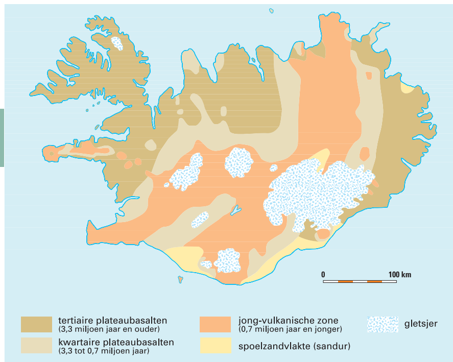
Geologische kaart van IJsland
